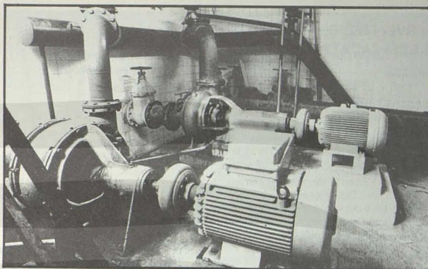
Emissari «Pi Rodó»
