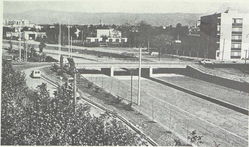
Perspectiva de la obra de encauzamiento de la Riera de Alforja ya terminada.
