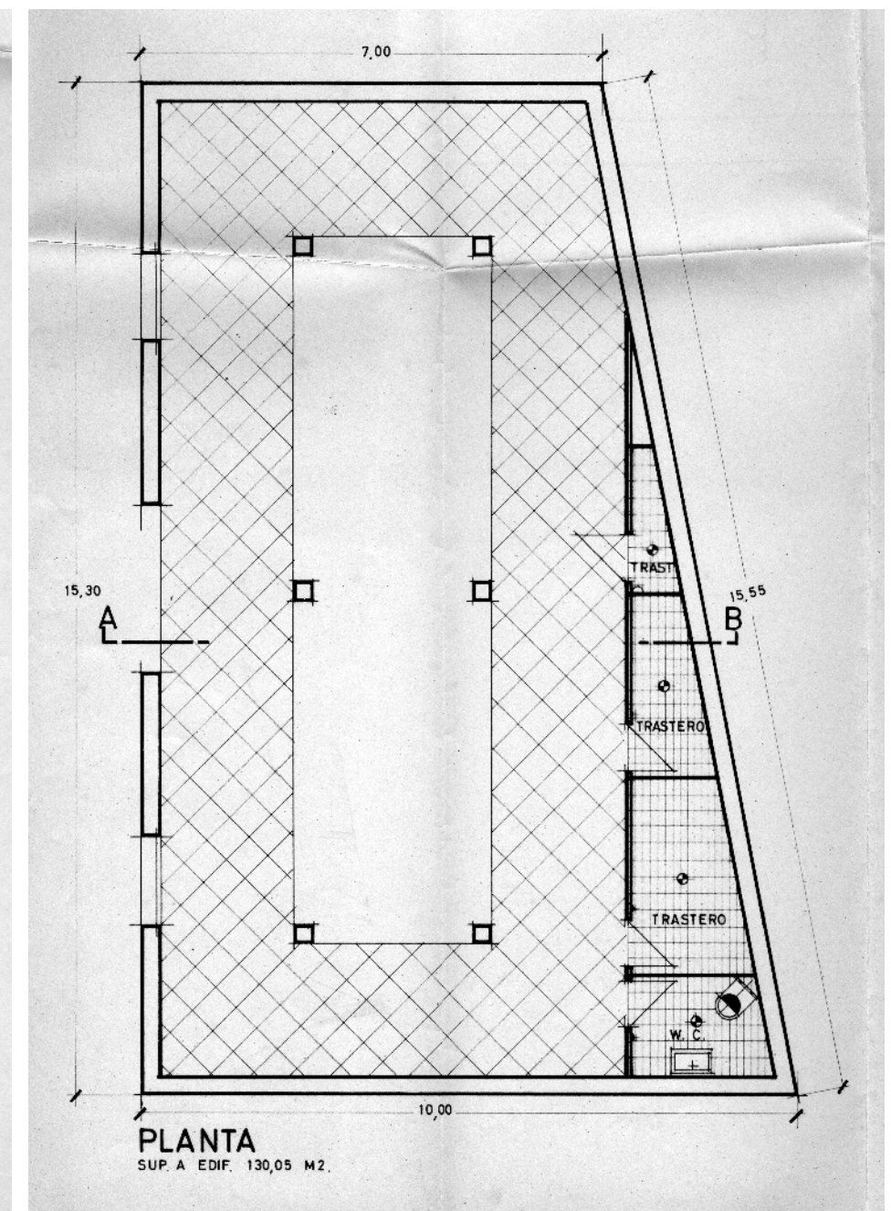
Plànol del projecte d'uns rentadors (1966)
